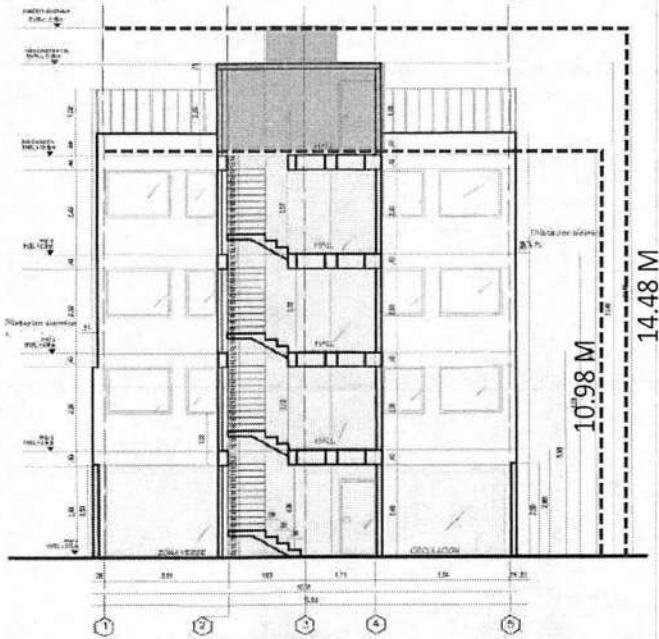
PLANOS ARQUITECTÓNICOS 2 / 2 A – APROBADOS EN LA LC 11001-1-20-3080
