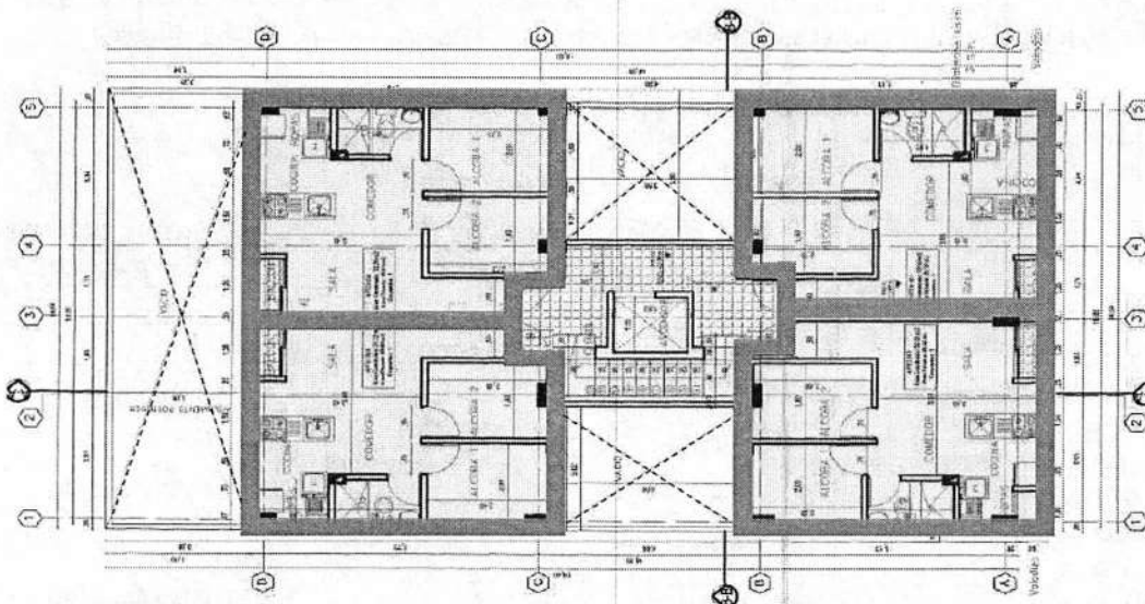
PLANOS ARQUITECTÓNICOS 1 / 2 A – APROBADOS EN LA LC 11001-1-20-3080
