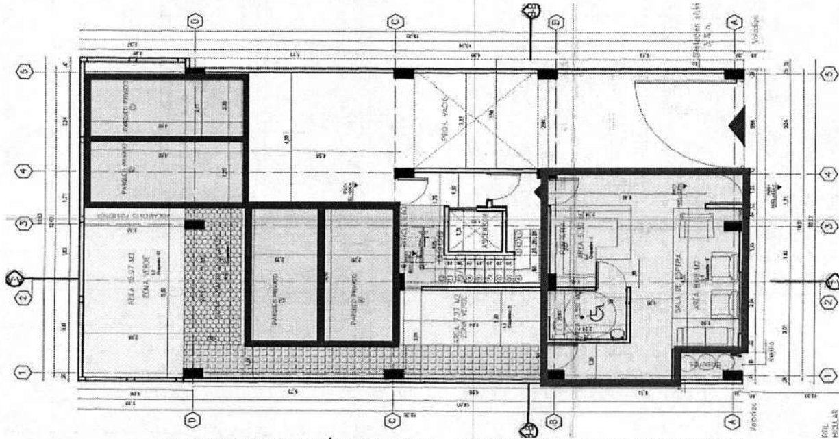
PLANOS ARQUITECTÓNICOS 1 / 2 A – APROBADOS EN LA LC 11001-1-20-3080
