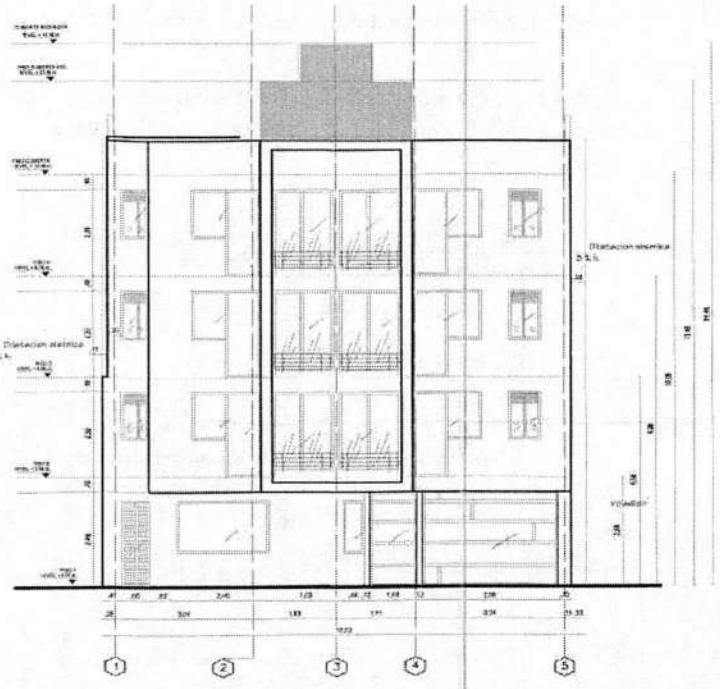
PLANOS ARQUITECTÓNICOS 2 / 2 A – APROBADOS EN LA LC 11001-1-20-3080
