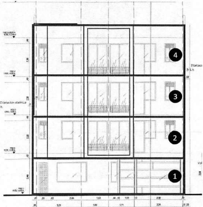
FACHADA APROBADA EN LA LC 11001-1-20-3080
